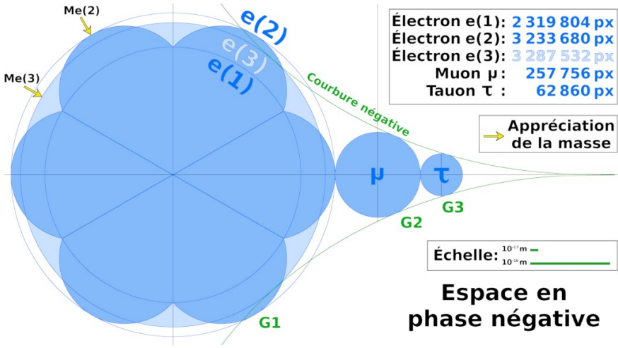
Tab 6.12 : Calcul graphique des masses des leptons de charge négative -1
