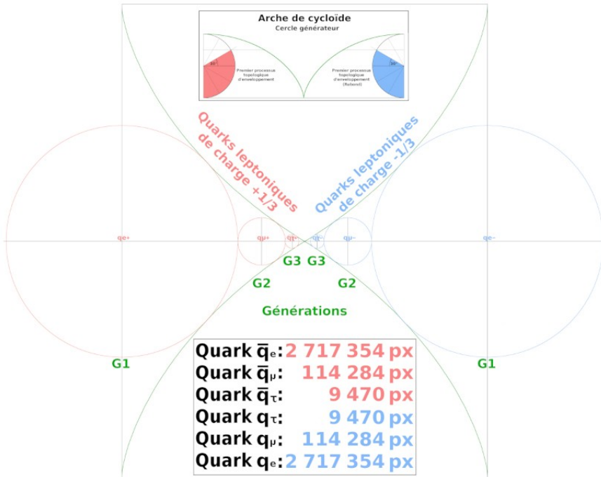
Fig. 6.16 : Quarks leptoniques « libres » - Création d'une paire électron / positon
