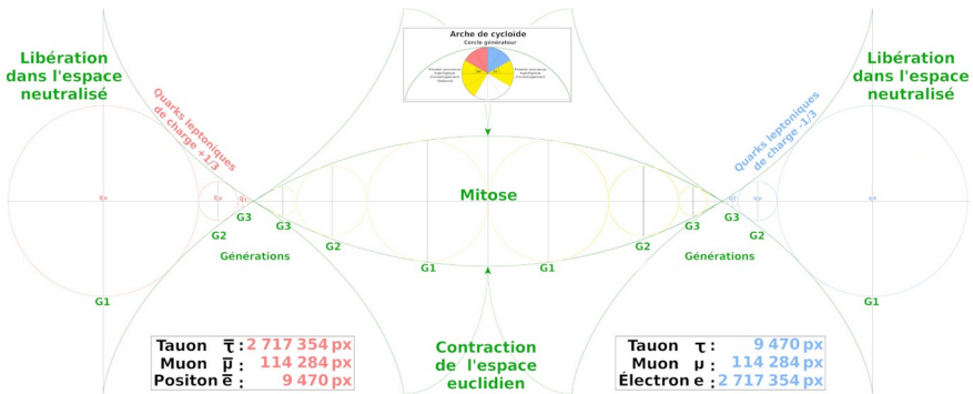
Fig. 6.18 : Processus topologique de simple enveloppement – Création de paire
