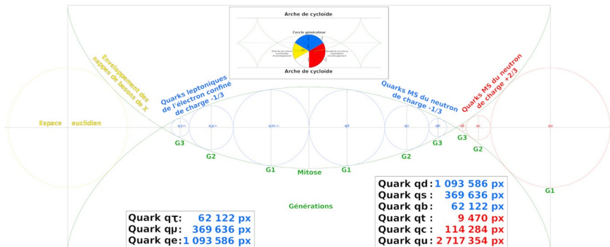
Fig. 6.17 : Processus topologique de double enveloppement – Genèse d'un neutron
